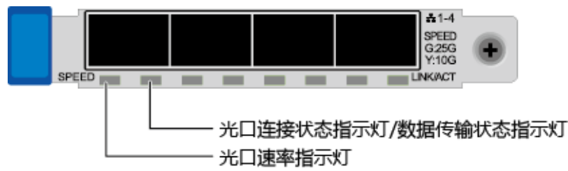
图4-13 TM280（4*25GE/10GE 光口）
