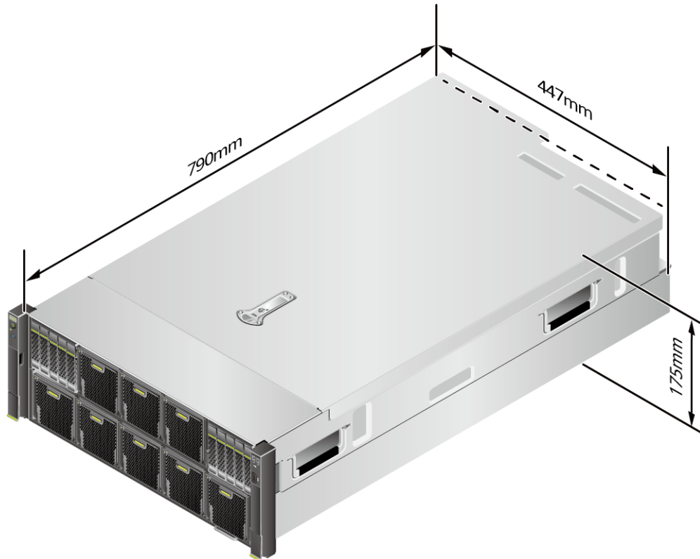
图5-1 物理尺寸
