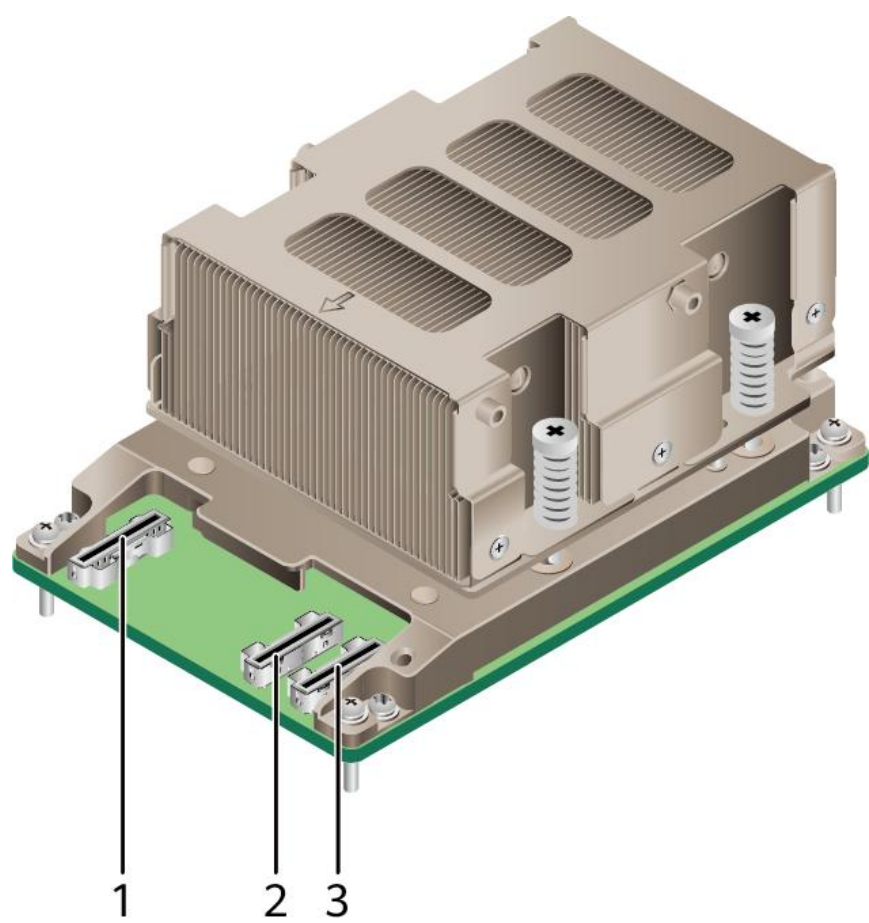
图4-17 NPU 模组接口示意图
