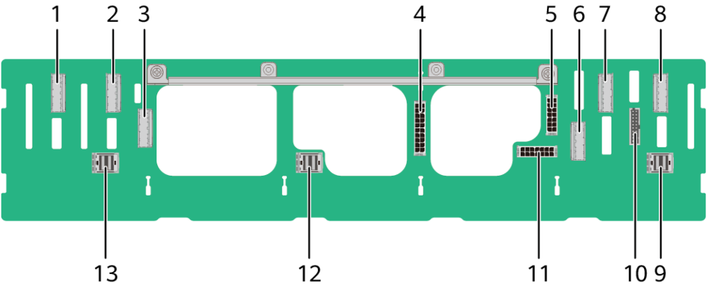
图4-15 硬盘背板
