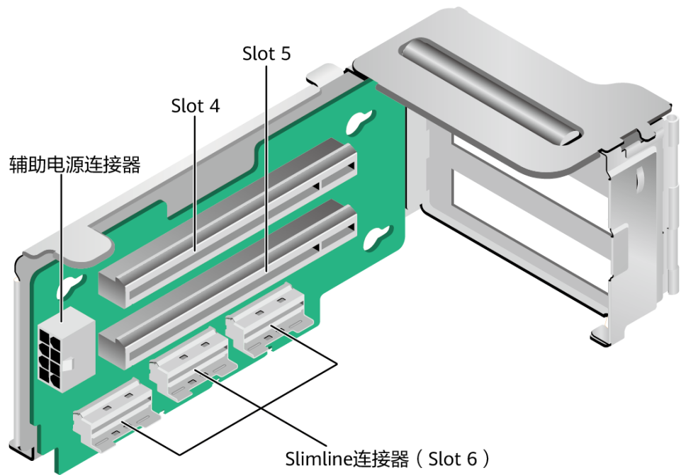
图4-12 Riser 卡 2 示意图
