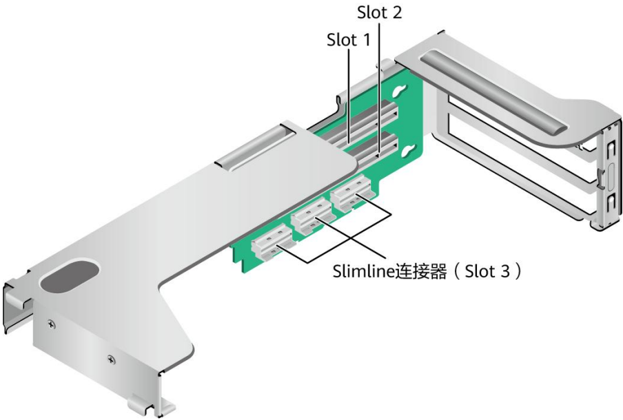
图4-11 Riser 卡 1 示意图
