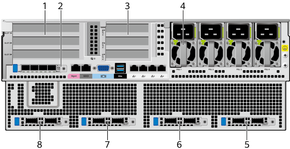
图4-3 后面板组件示意图
