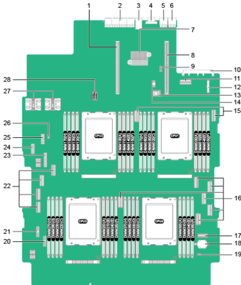
图4-16 主板接口
