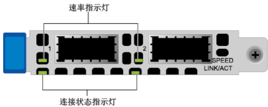
图4-14 参数面接口卡（2*200GE 光口）
