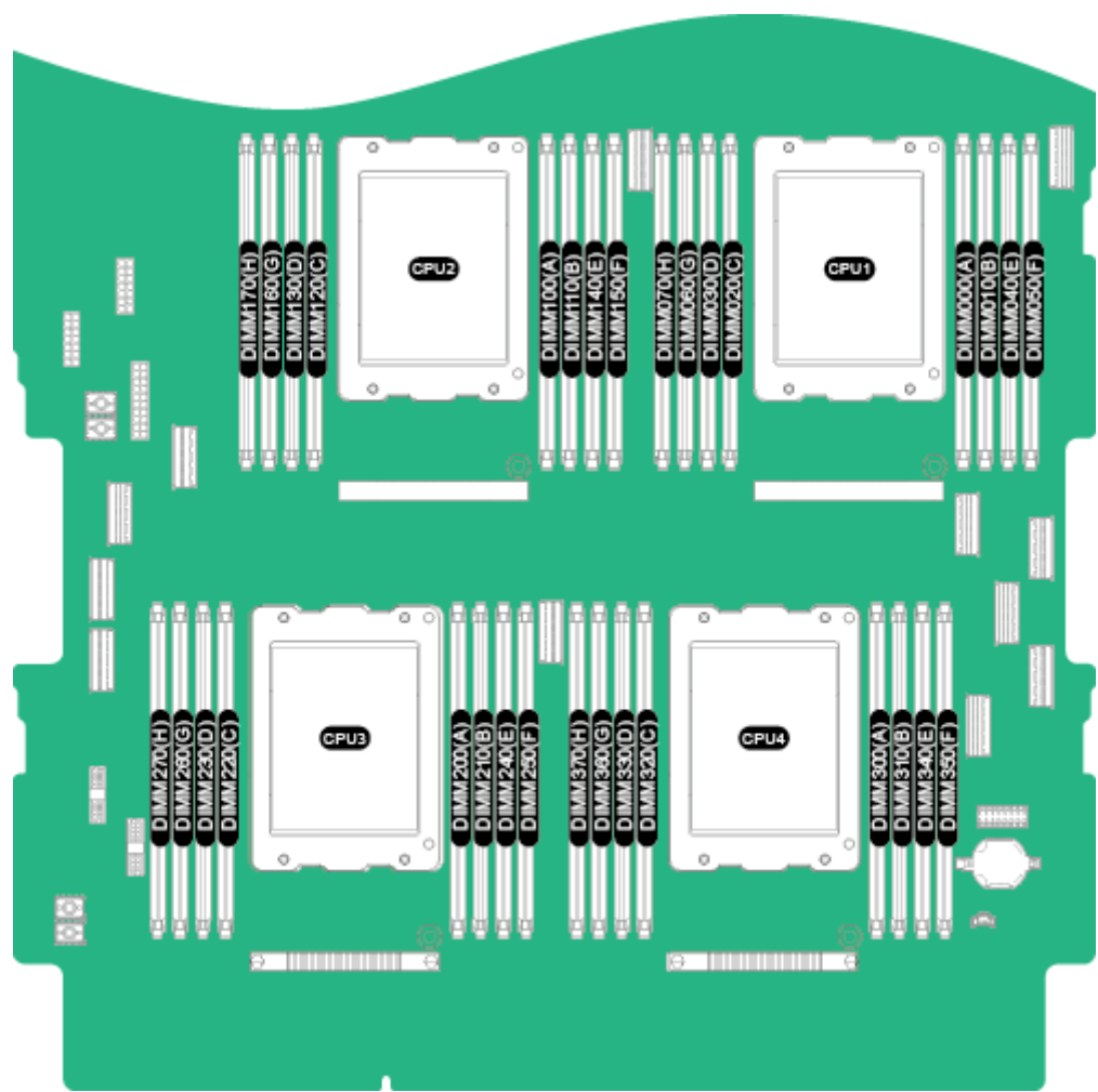
图4-20 内存槽位编号
