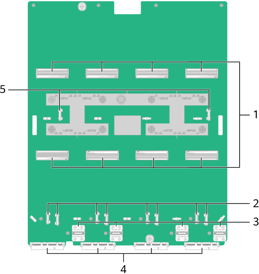
图4-18 NPU 载板接口
