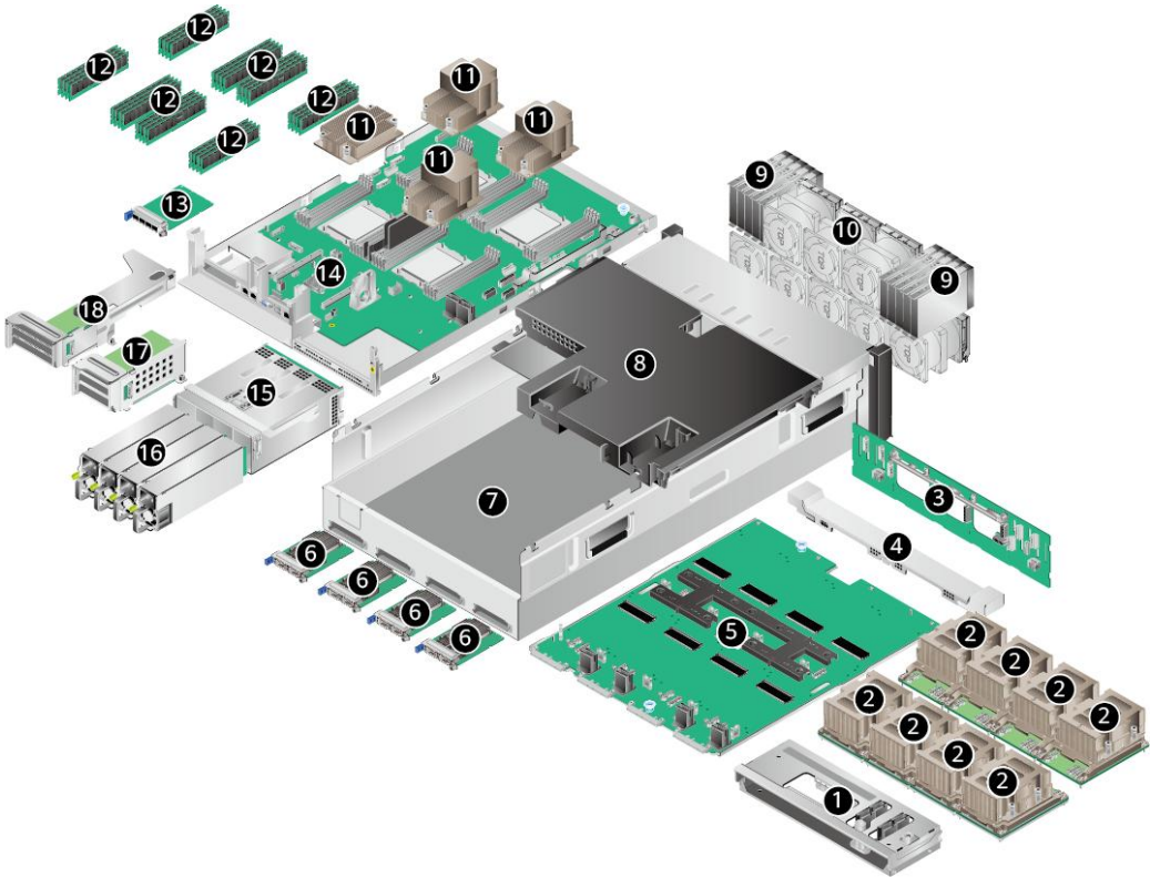
图3-1 部件示意图
